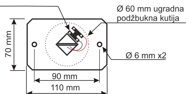
Detalj montaže
